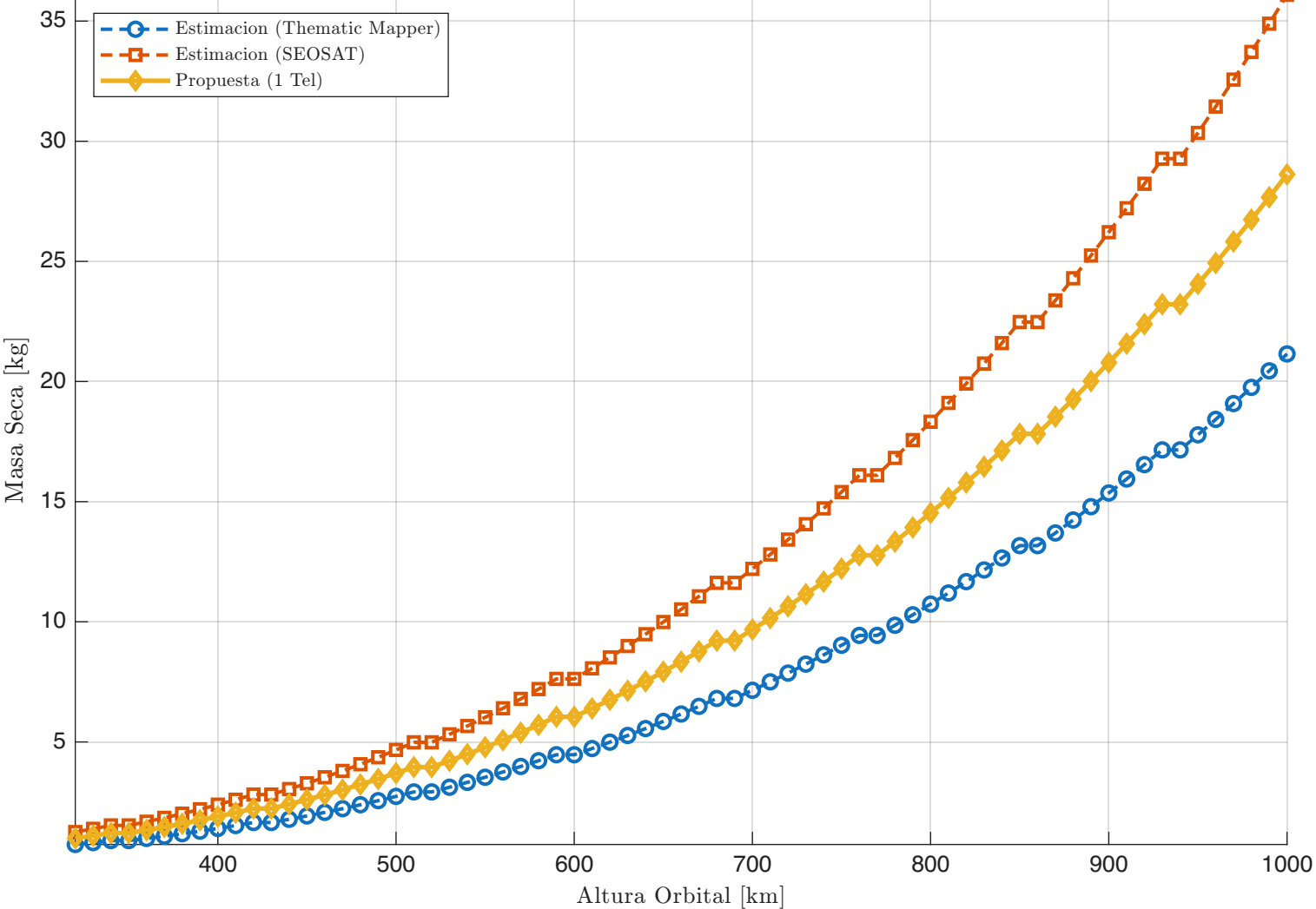
Comparativa de Masa Seca vs. Altura Config: 1 Sat, 1 Tel, Det 3, Korsch
